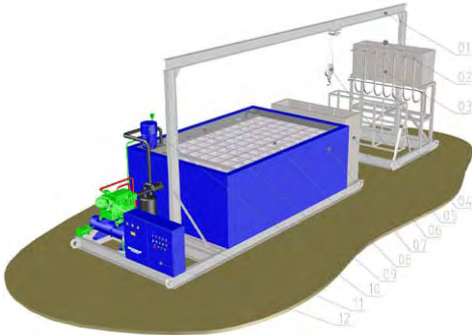
01 导轨， 02 加水箱， 03 加水机构， 04 倒冰架， 05 起吊装置， 06 融冰池， 07 盐水池， 08 制冰桶， 09 钛盘管蒸发器， 10 盐水搅拌机， 11 制冷机组， 12 电控箱
